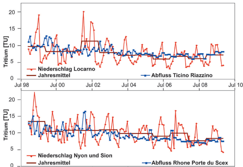
Abb. 2 Tritiumkonzentrationen im Niederschlag in Locarno und gemittelte Konzentrationen der beiden Stationen Nyon und Sion im Vergleich zu jenen im Ticino in Riazzino und in der Rhone in Porte du Scex. Die Tritiumkonzentrationen im Ticino liegen über dem Mittel der Niederschläge, jene in der Rhone dagegen darunter.
