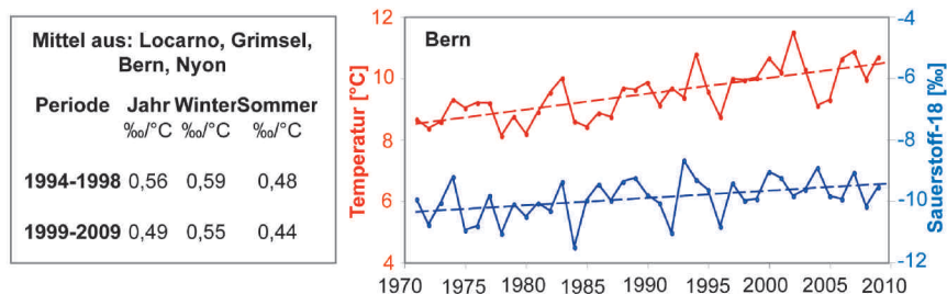
Abb. 4 Mittlerer Temperaturfaktor von \delta^{18}\text{O} an ausgewählten ISOT-Niederschlagsstationen (links) und Trend von Temperatur und Sauerstoff-18 in den Jahresmitteln der letzten 40 Jahre in Bern (rechts).
