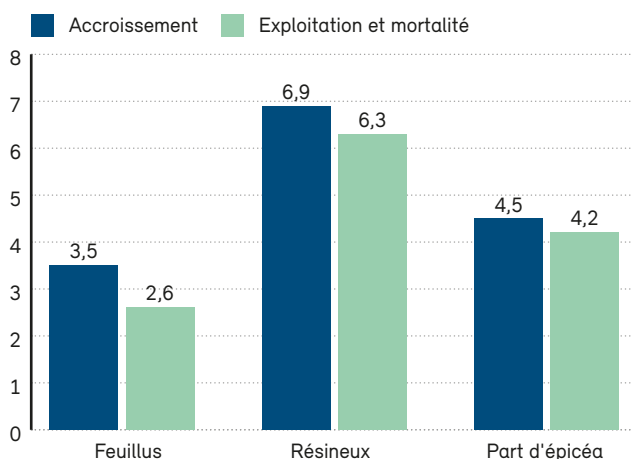
Graphique 3.3 : Accroissement, exploitation, mortalité par essence, IFN3-IFN4 1
